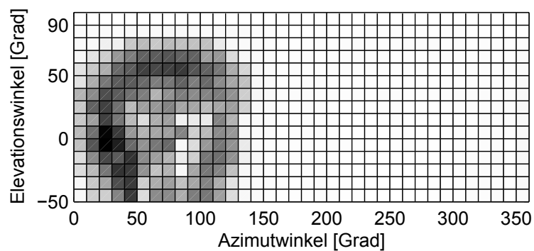
Abbildung 2.27: Lokalisationsmatrix mit Kopfdrehung = -20^\circ und Schallquelle = 20^\circ bezogen auf das Referenzsystem (Kopfdrehung = 0^\circ )
