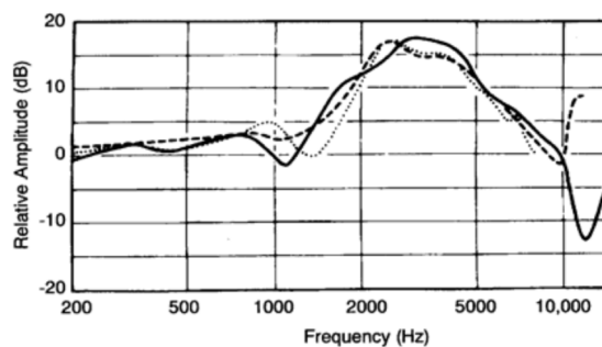
Abbildung 1.5: Übertragungsfunktion des Außenohrs bei frontal platzierter Schallquelle [Gel97]
