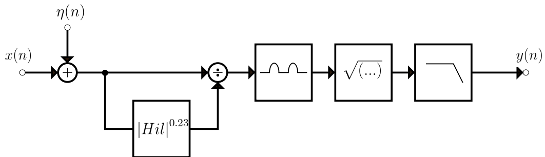
Abbildung 2.6: Signalflussplan des neuronalen Übertragungspfad
