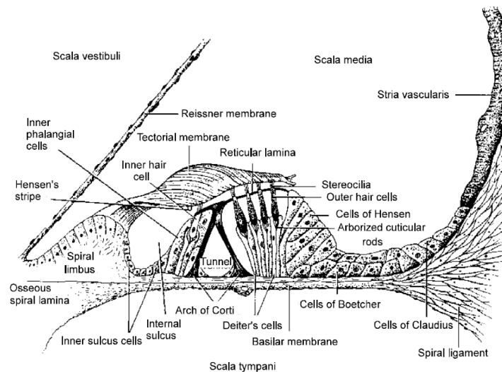
Abbildung 1.10: Stark vergrößerte Darstellung eines Cochleaerschnittes [GGF89]
