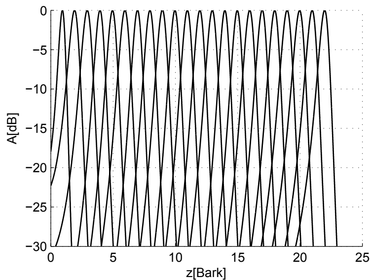
Abbildung 2.5: Übertragungsfunktionen aller 22 Barkbandfilter
