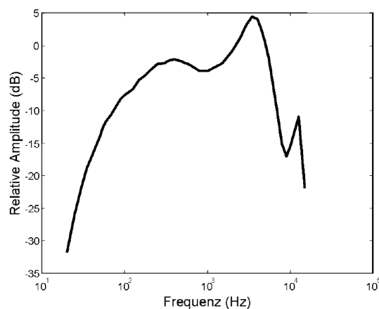
Abbildung 1.7: Übertragungsfunktion des Außenohrs und Mittelohrs [Lab06]
