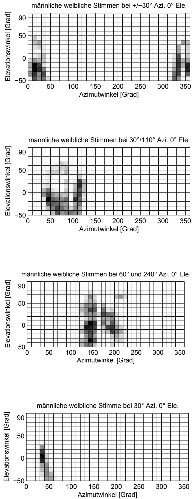
Abbildung 3.12: 2 nichtkorrelierte Stimmen an unterschiedlichen Orten
