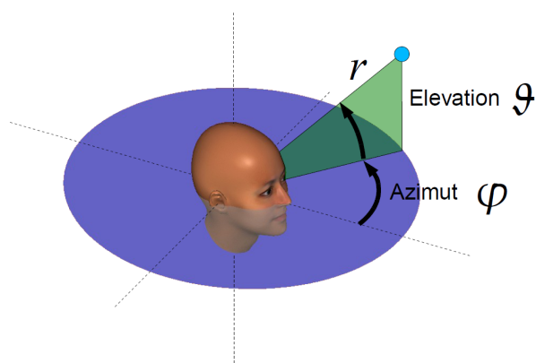
Abbildung 1.2: Position einer Schallquelle [Maj10]
