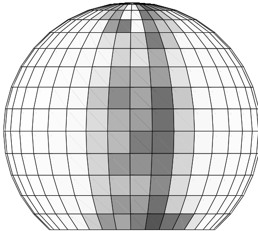
Abbildung 3.21: Phantomschallquelle bei 0^\circ Azimut in frontaler Kugeldarstellung
