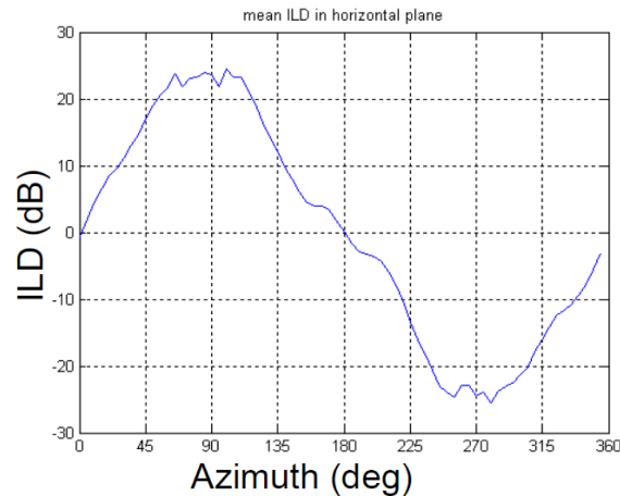
Abbildung 1.15: Durchschnittliche Pegeldifferenz abhängig vom Azimutwinkel gemessen an einem Kunstkopf [Maj10]
