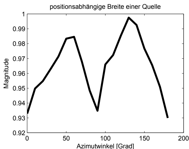
Abbildung 2.32: Quellenbreite einer Schallquelle bei unterschiedlichen Positionen
