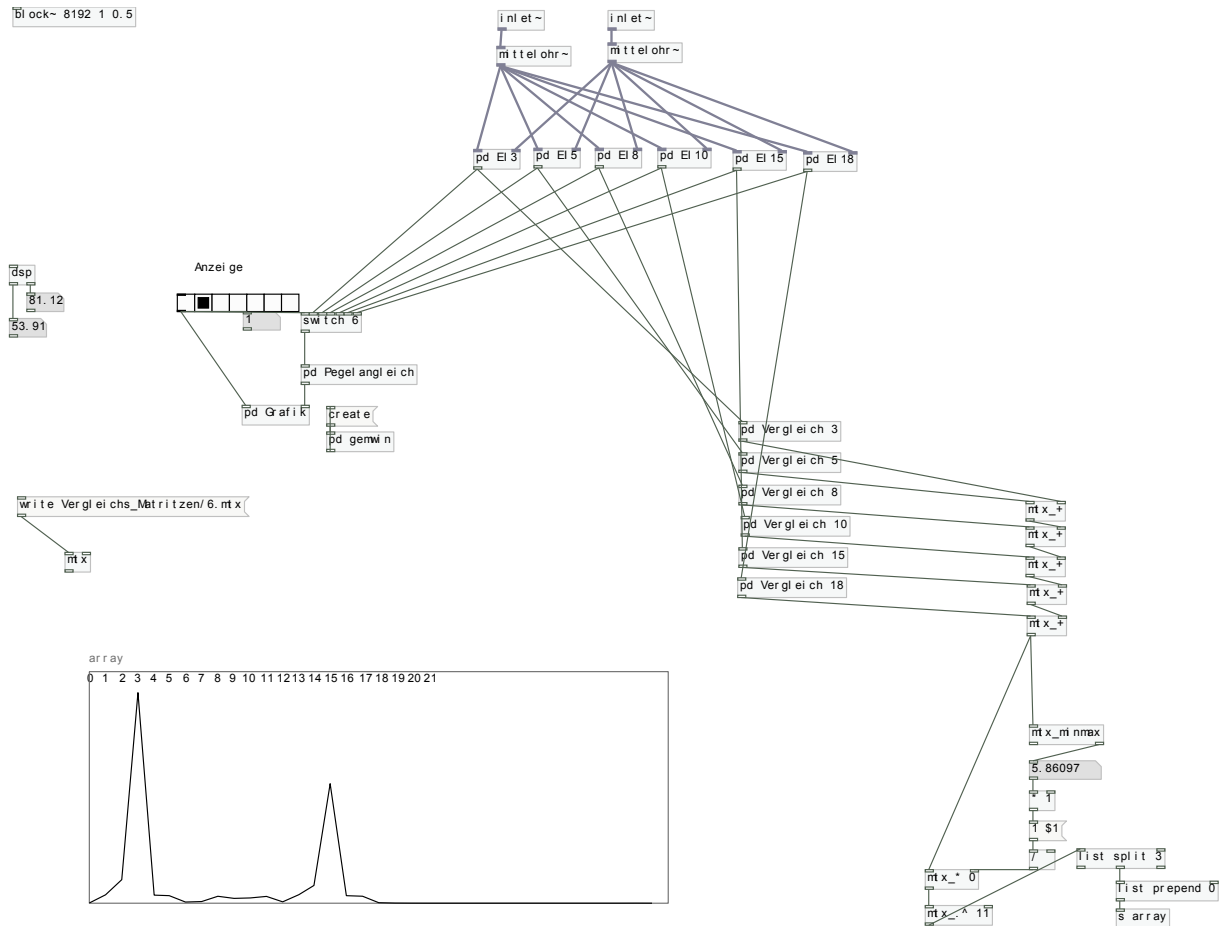
Abbildung 2.36: Ansicht eines Teils des Echtzeit-Lokalisationsmodells in Pd; links unten im Bild wird eine Schallquelle bei 30° lokalisiert
