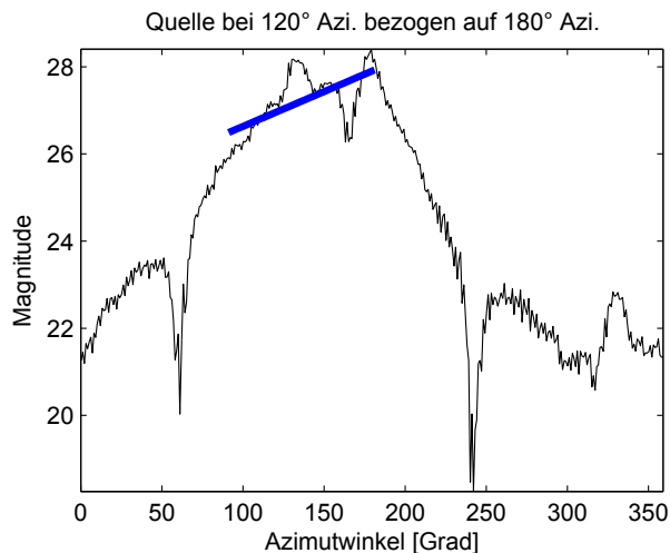
Abbildung 2.31: Lokalisationsvektor einer Quelle bei 120° mit angeglichenen Geraden
