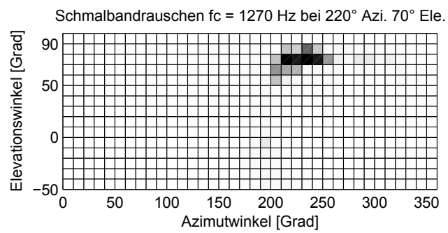
Abbildung 3.4: Schmalbandrauschquelle bei unterschiedlichen Mittenfreq. und Winkeln
