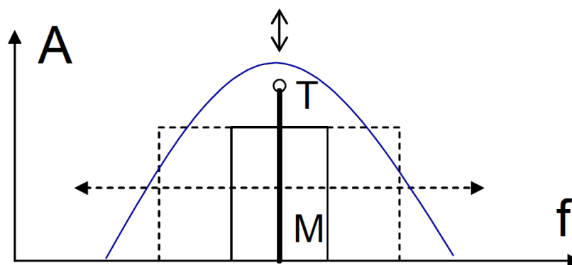
Abbildung 1.13: Bestimmung der Mithörschwelle: Testsignal mit variablen Pegel bei Mittenfrequenz eines Schmalbandrauschens mit variabler Bandbreite [Lab06]
