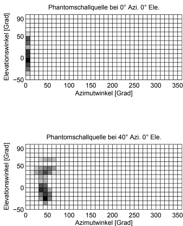
Abbildung 3.9: Phantomschallquellen bei 0^\circ und 40^\circ Azimutwinkel
