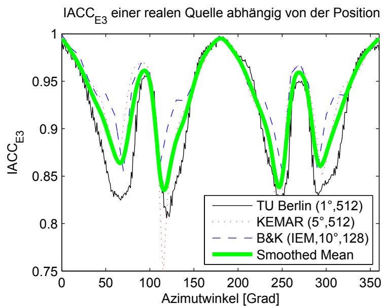
Abbildung 1.22: Berechnung der IACC_{E3} abhängig von der Quellenposition von Matthias Frank
