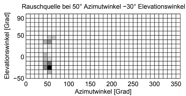
Abbildung 3.1: Lokalisationsmatrizen einer Rauschquelle bei unterschiedlichen Winkeln
