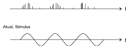
Abbildung 1.11: Phase Locking der Neuronen: Spikes synchron zur Phase der oberen Halbwellen (oben) akustischer Stimulus (unten) [Lab06]
