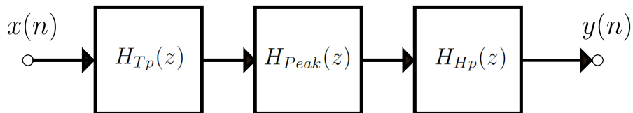
Abbildung 2.3: Signalflussplan für das Außen- und Mittelohr
