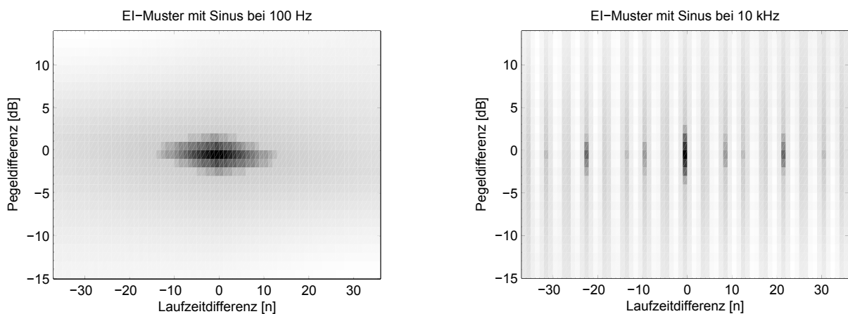
Abbildung 2.13: EI-Muster mit Sinustönen bei 100 Hz und 10000 Hz
