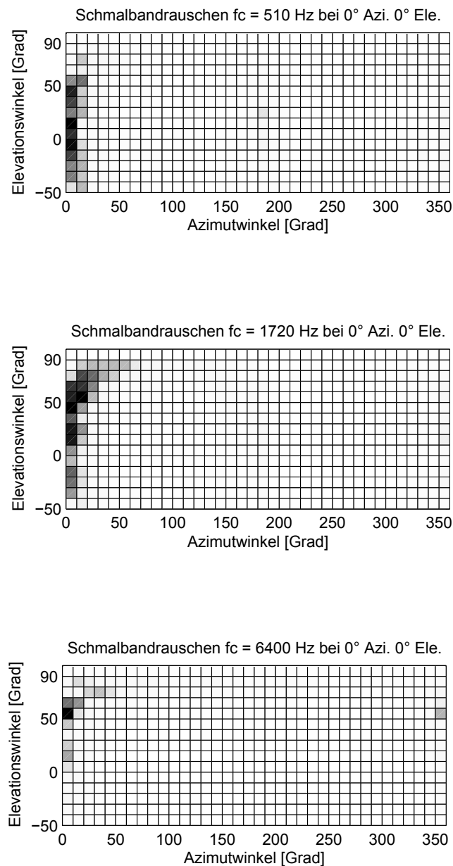
Abbildung 3.3: Schmalbandrauschquelle bei unterschiedlichen Mittenfrequ. und 0^\circ Azimut
