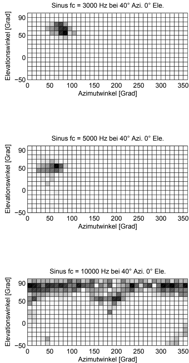
Abbildung 3.6: Sinusquelle mit 3000Hz, 5000 Hz und 10000 Hz bei 40° Azimut
