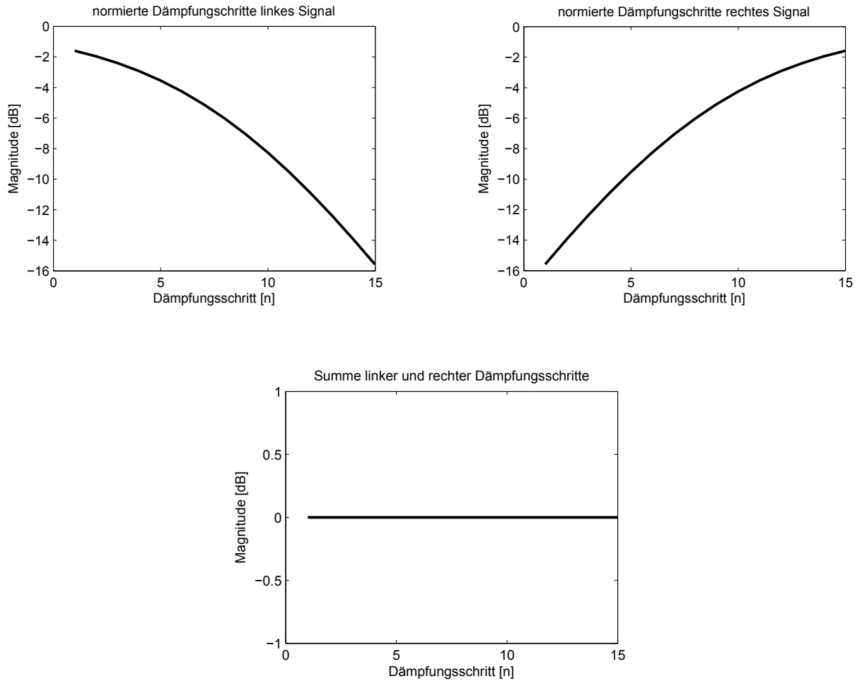
Abbildung 2.11: Verlauf der Dämpfungsschritte für linkes und rechtes Signal
